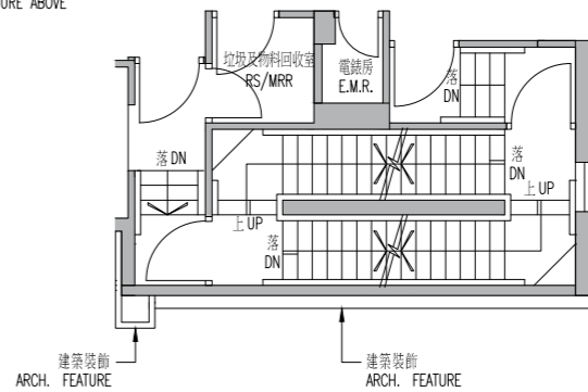
32/F Unit A Part Plan 32樓之部分平面圖
