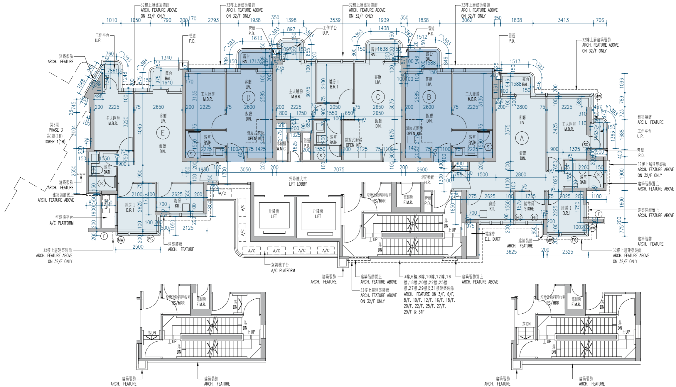
31/F Unit A Part Plan 31樓之部分平面圖
